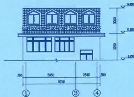
①~④轴局部立面图 (变更后) 1:100
