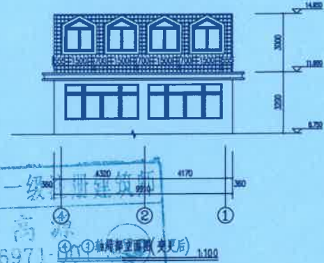
④~①轴局部立面图 (变更后) 1:100
