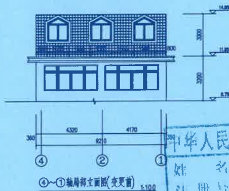
④~①轴局部立面图 (变更前) 1:100
