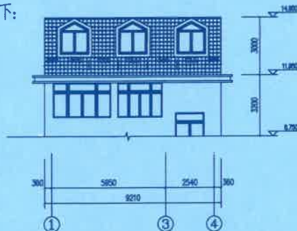
①~④轴局部立面图 (变更前) 1:100
